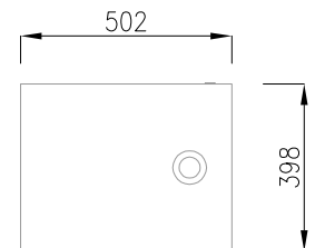
půdorys | 1: 20
